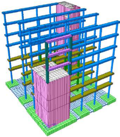
Vista del modello di calcolo FEM: a sinistra Fabbricato H, a destra Palazzina Uffici / View of the FEM calculation model: Building H on the left, Office Building on the right
