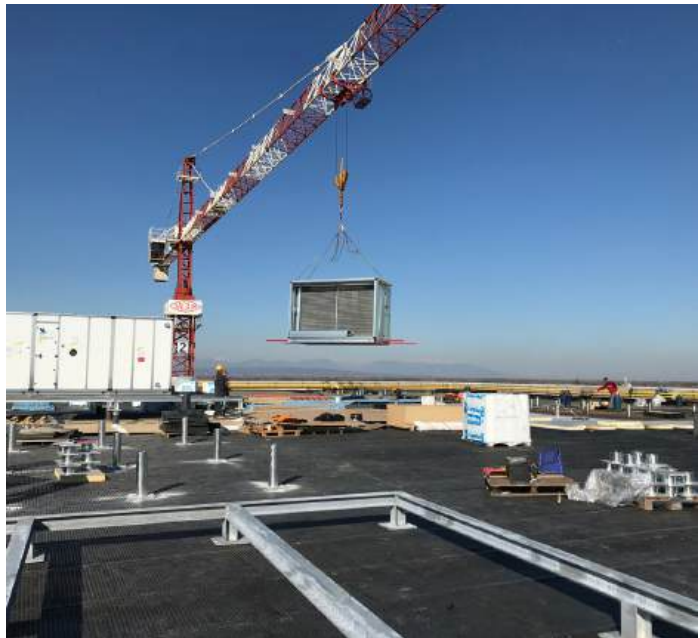
Installazione delle UTA in copertura / Installation of AHUs on the roof
