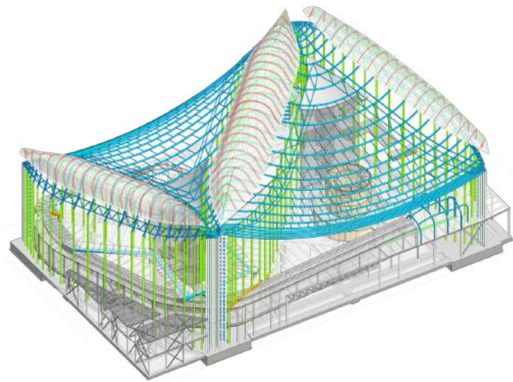
Modello tridimensionale strutturale - software Revit / Three-dimensional structural model - Revit software
