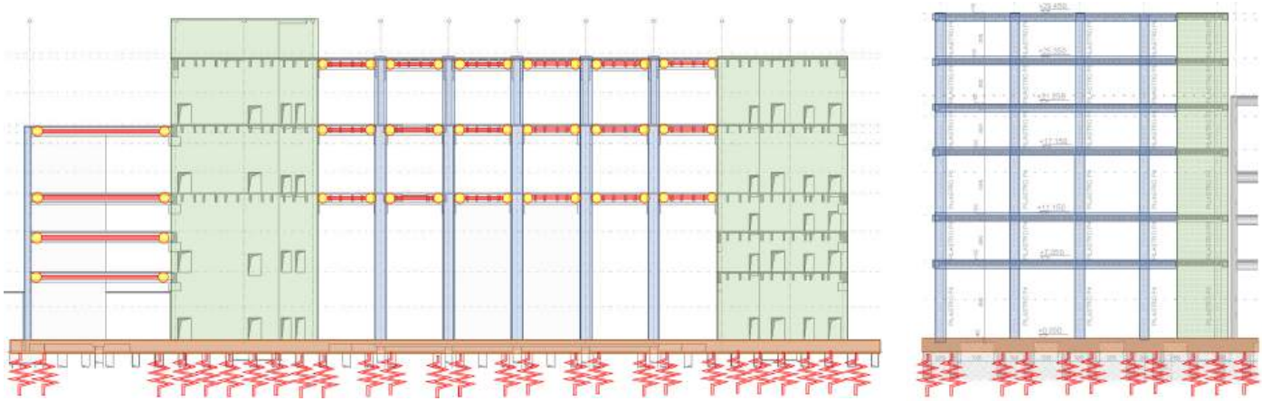
A sinistra: schema statico Fabbricato H - A destra: schema statico Palazzina Uffici / Left: static diagram of Building H - Right: static diagram of Office Building
