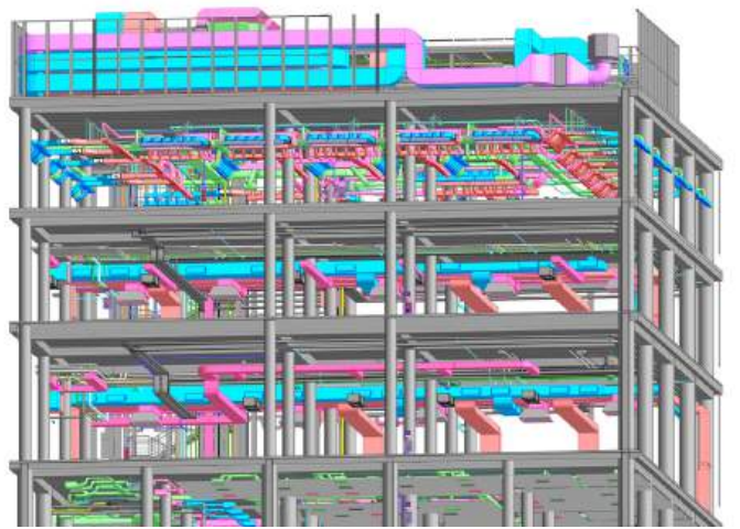
Assonometria dal modello BIM degli impianti in copertura / Axonometric projection from the BIM model of the roof systems
