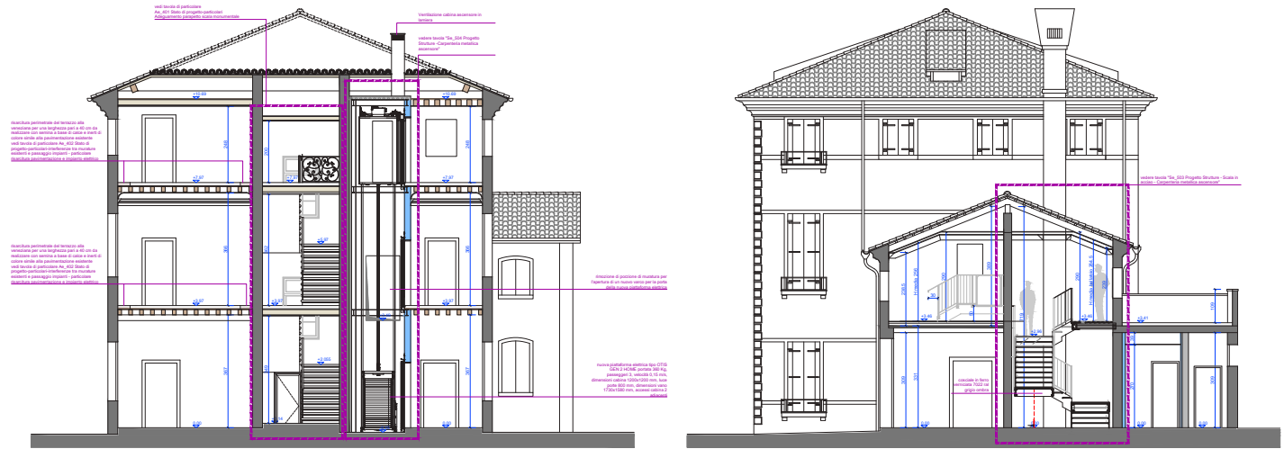
Stato di progetto - sezioni - simulazione intervento / Project status - sections - intervention simulation
