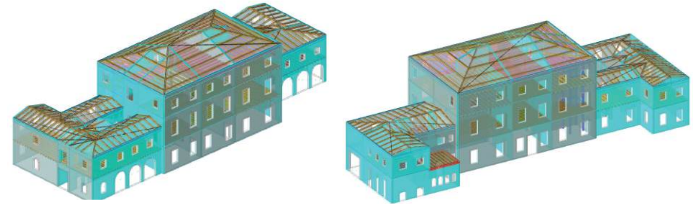
Modelli di calcolo / Calculation models
