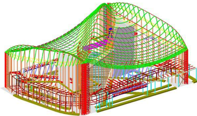
Modello di calcolo agli elementi finiti - software MIDAS GEN / Finite element analysis model - MIDAS GEN software
