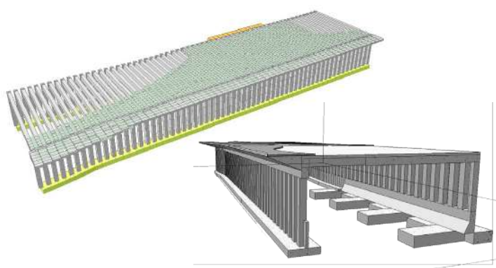
Modelli BIM della galleria / BIM models of the tunnel
