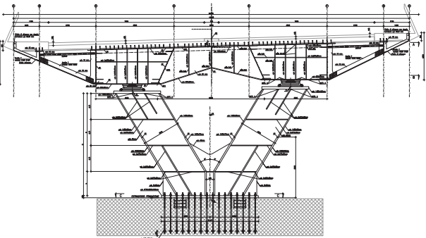
Sezione strutturale tipologica del viadotto principale / Typological structural section of the main viaduct
