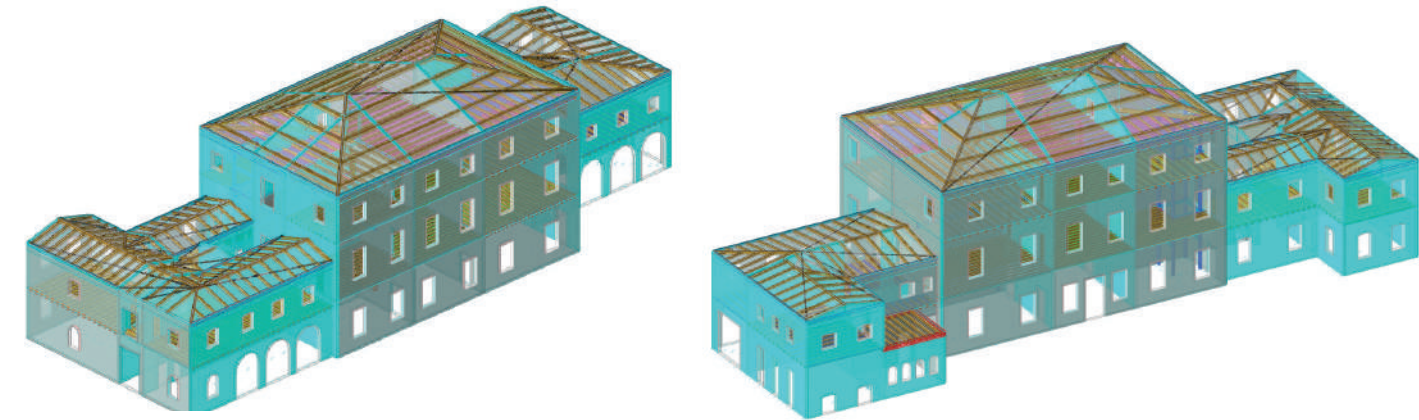
Modelli di calcolo / Calculation models
