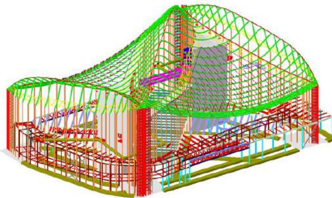
Modello di calcolo agli elementi finiti - software MIDAS GEN / Finite element analysis model - MIDAS GEN software
